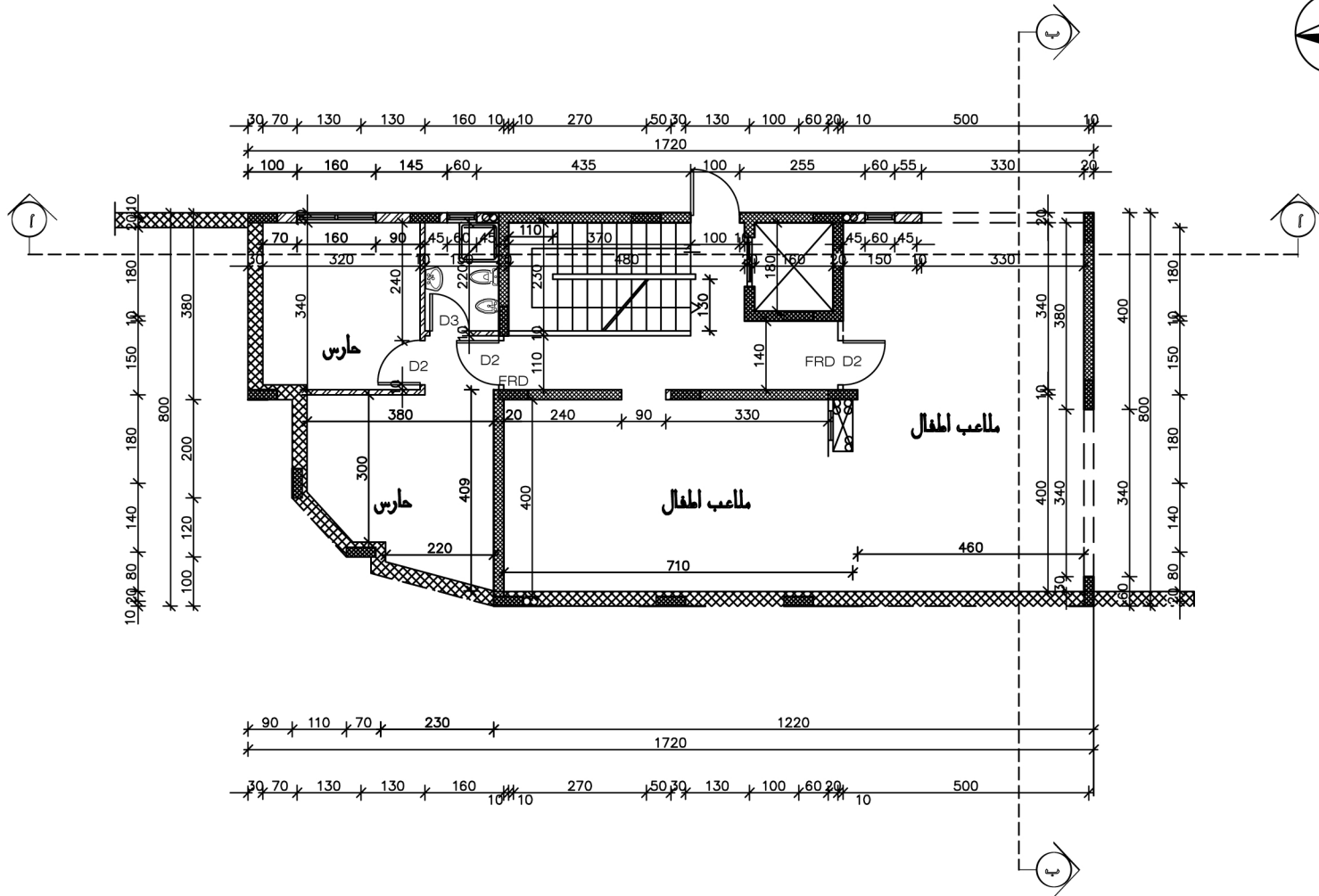
مخطط الطابق التسوية
