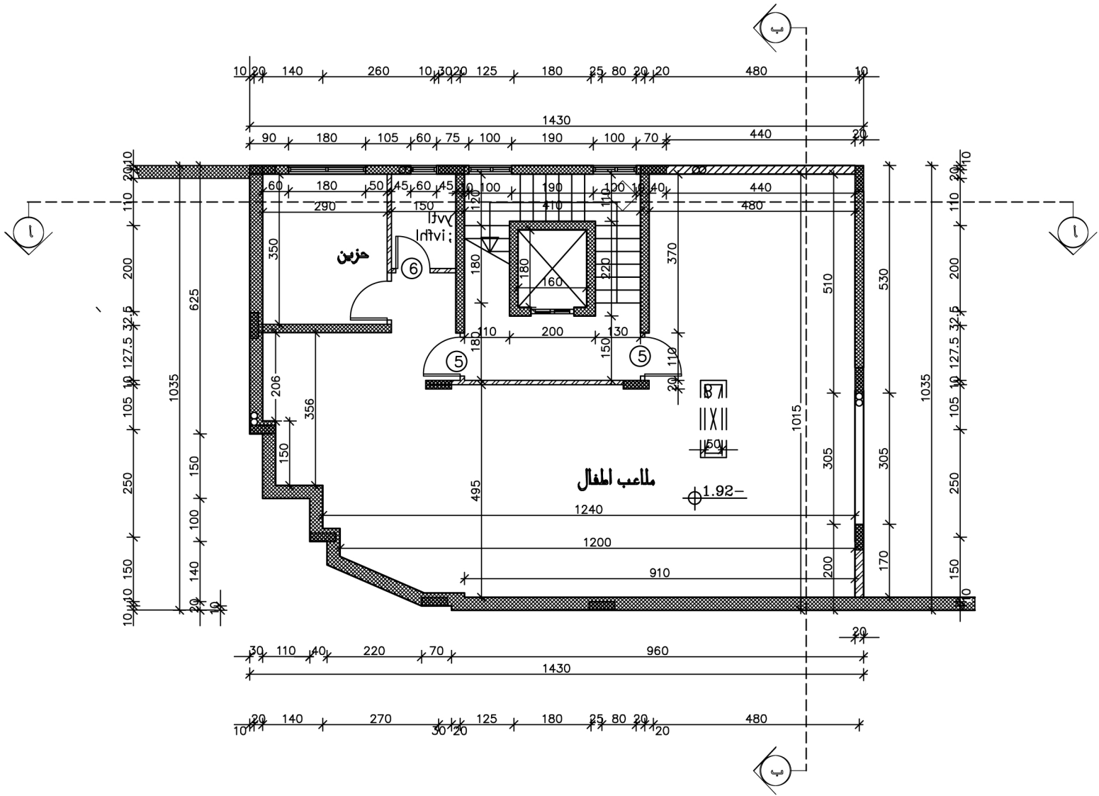
مخطط الطابق التسوية
