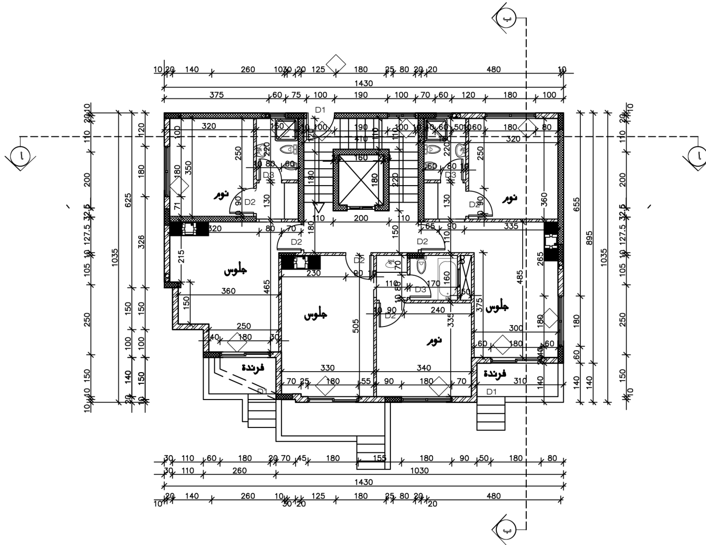
مخطط الطابق الارضى
